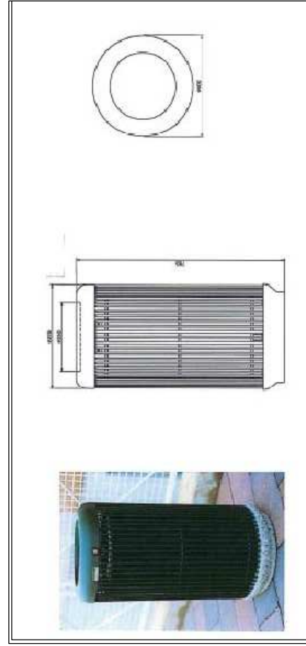
particolare cestone
