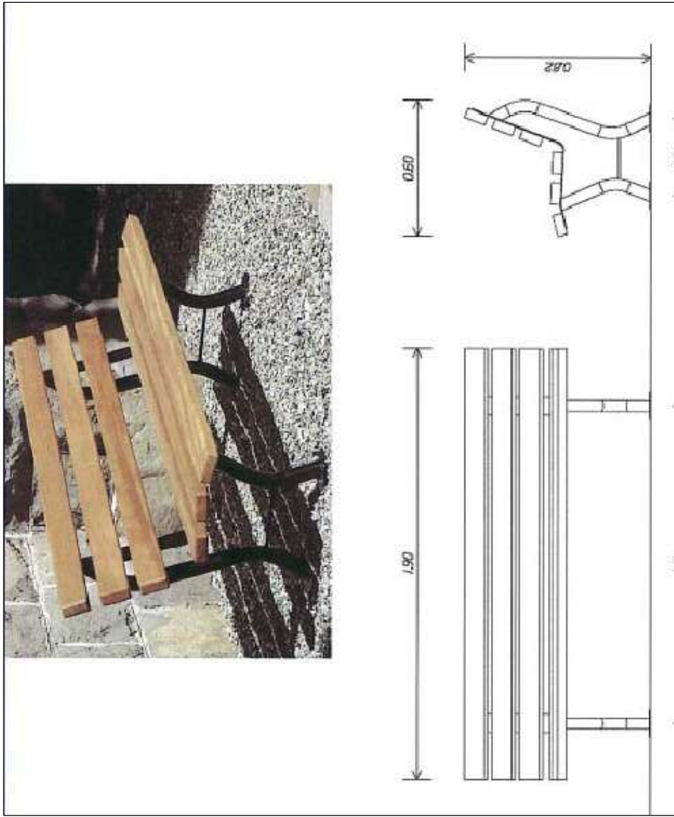
particolare panchine
